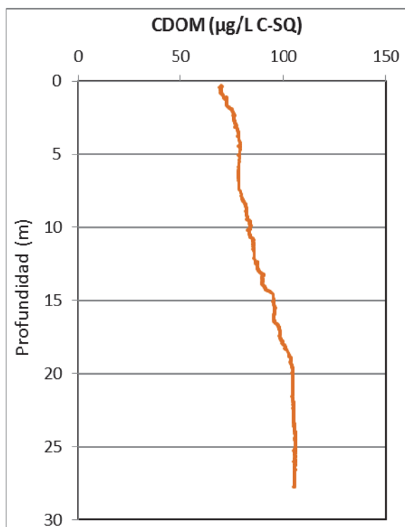
Figura 5. Perfil vertical de la conductividad y de la materia orgánica cromofórica.
